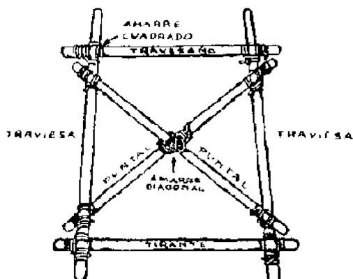
Un puente sencillo puede ser construido con dos caballetes. El diagrama muestra el arreglo de las dos partes. Todos los amarres son cuadrados, excepto el del centro de los palos cruzados.
